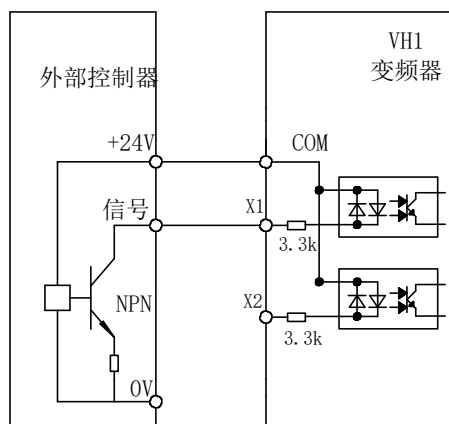
使用外部24V电源的漏型接线方法
