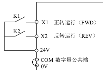
PNP型接法
