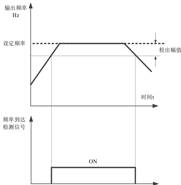
一段速曲线
