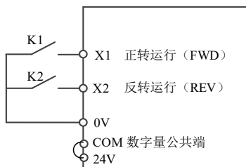
NPN型接法
