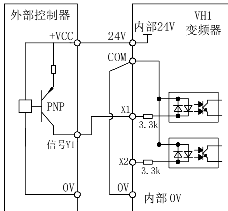
使用变频器内部24V电源的源型接线方法
