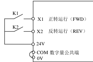
PNP型接法
