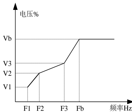
注：V1~V3：多点 VF 曲线第 1~3 段电压百分比 F1~F3：多点 VF 曲线第 1~3 段频率点
