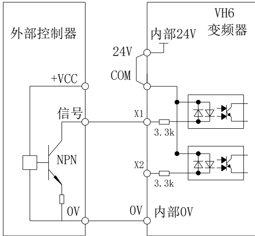
使用扩展卡上24V电源的漏型接线方法
