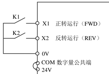
NPN型接法
