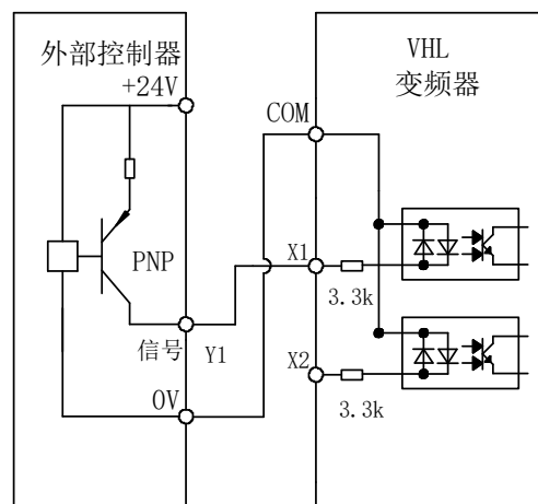
使用外部24V 电源的源型接线方法
