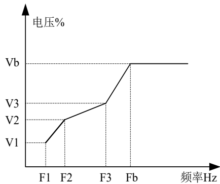
V1~V3：多点 VF 曲线第 1~3 段电压百分比；F1~F3：多点 VF 曲线第 1~3 段频率点
