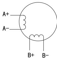
四线电机
