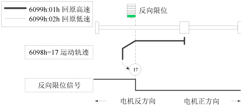
使用反向限位信号回原
