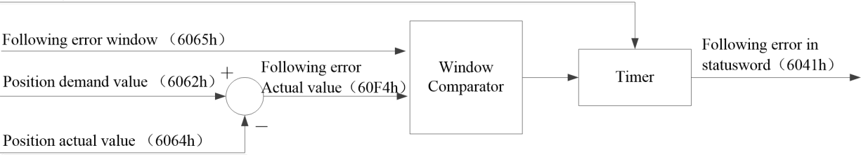
跟随误差功能示意图
