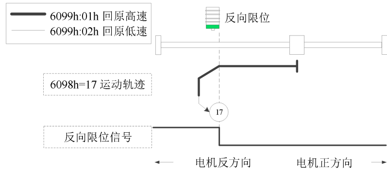
使用反向限位信号回原
