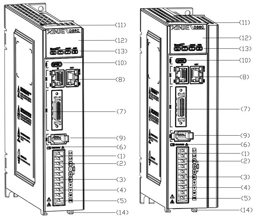
a) 驱动器 0. 1~0. 4kW 部件说明示意图 b) 驱动器 0. 75kW 部件说明示意图
