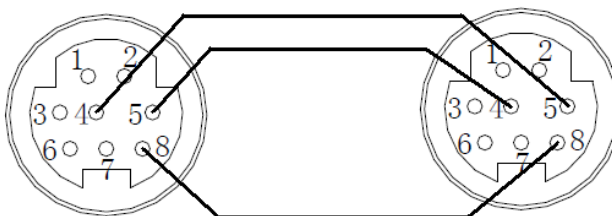
Mini Din 8 芯插座（孔）
