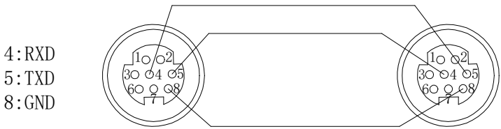
Mini Din8插座（孔）
