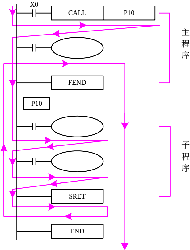
子程序执行图示说明：
