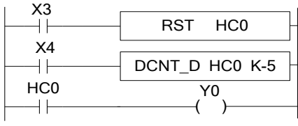
图 2（掉电保持减计数寄存器）
