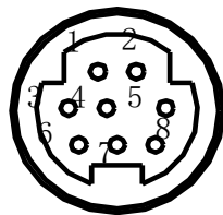
Mini Din 8 芯插座 (孔)
