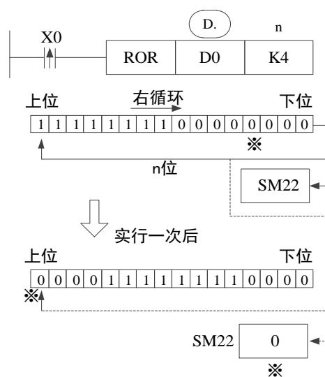
《循环右移》
