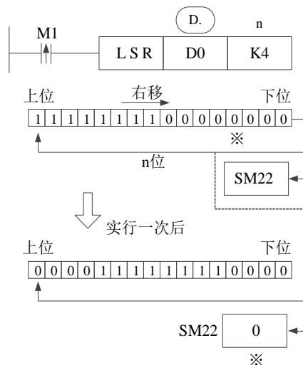
《逻辑右移》
