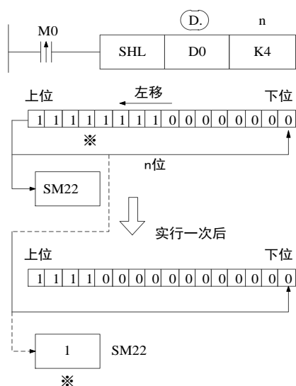
《算术左移》
