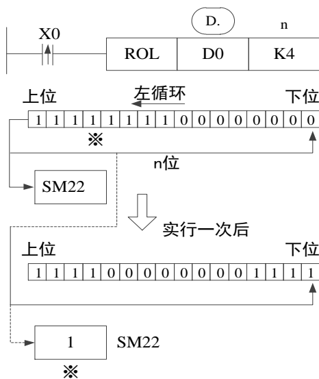
《循环左移》
