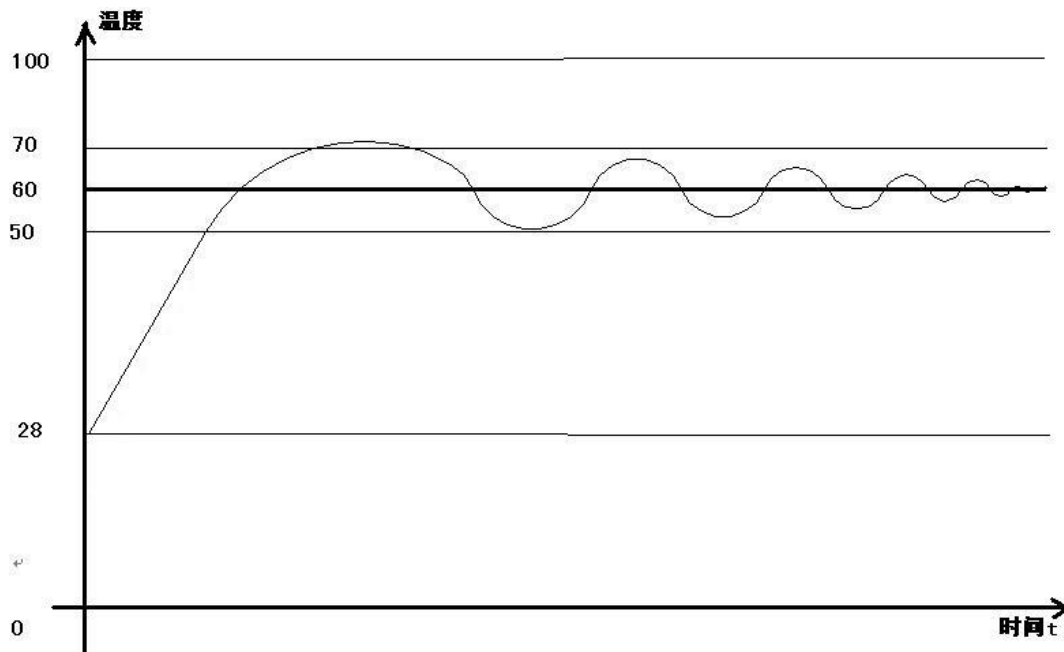
图 4 PID 自整定不允许超调波形图
