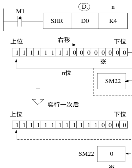
《算术右移》
