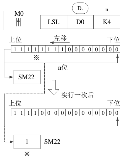
《逻辑左移》
