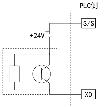
两线制（开或常闭）接近开关接线图示例
