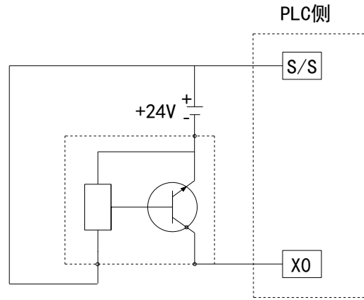
三线制（PN 型）接近开关接线图示例
