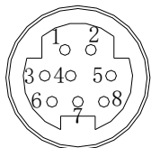
Mini Din 8 芯插座 (孔)
