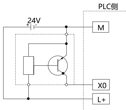
三线制（NPN 型）接近开关接线图示例
