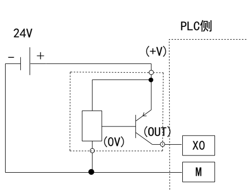
三线制接近开关接线图示例
