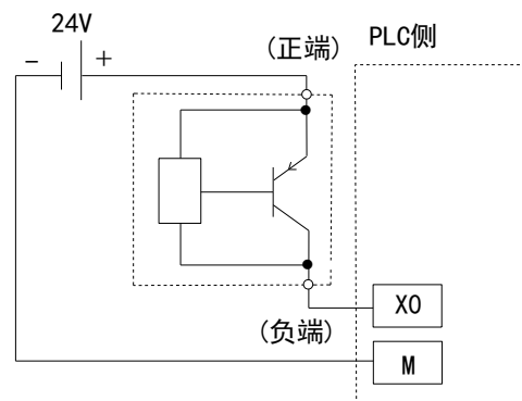
两线制接近开关接线图示例
