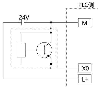
两线制（常开或常闭）接近开关接线图示例
