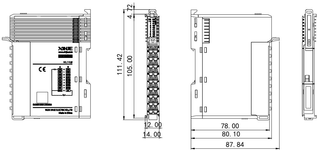
（单位：mm）
