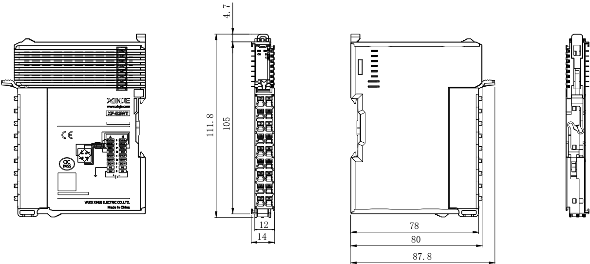
(单位: mm)
