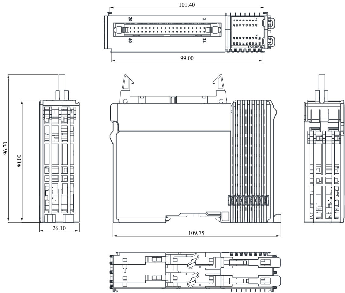
(单位：mm)
