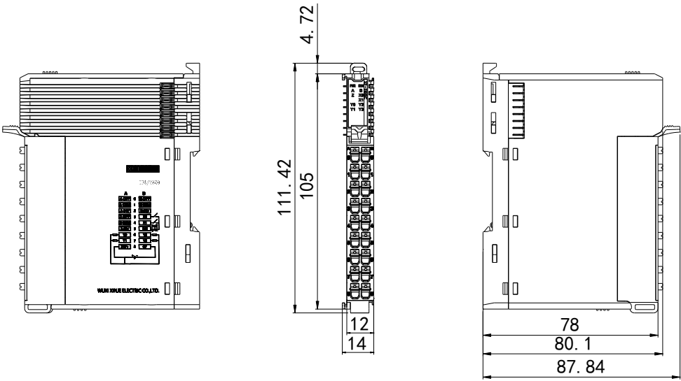
（单位：mm）
