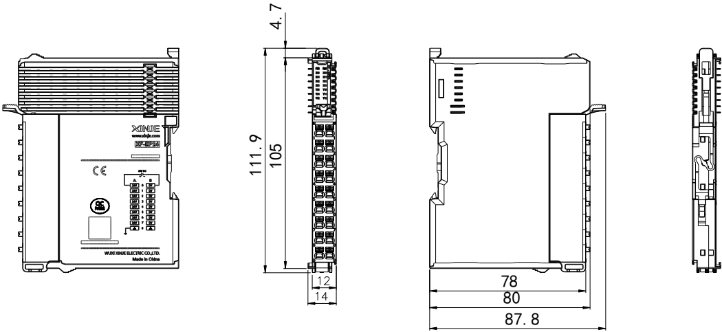
（单位：mm）
