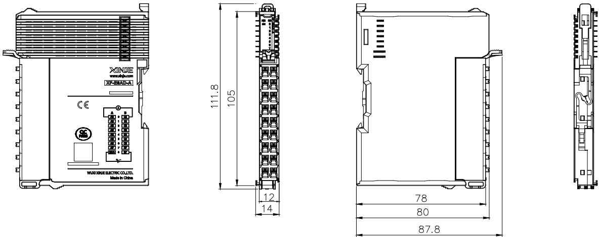
(单位：mm)
