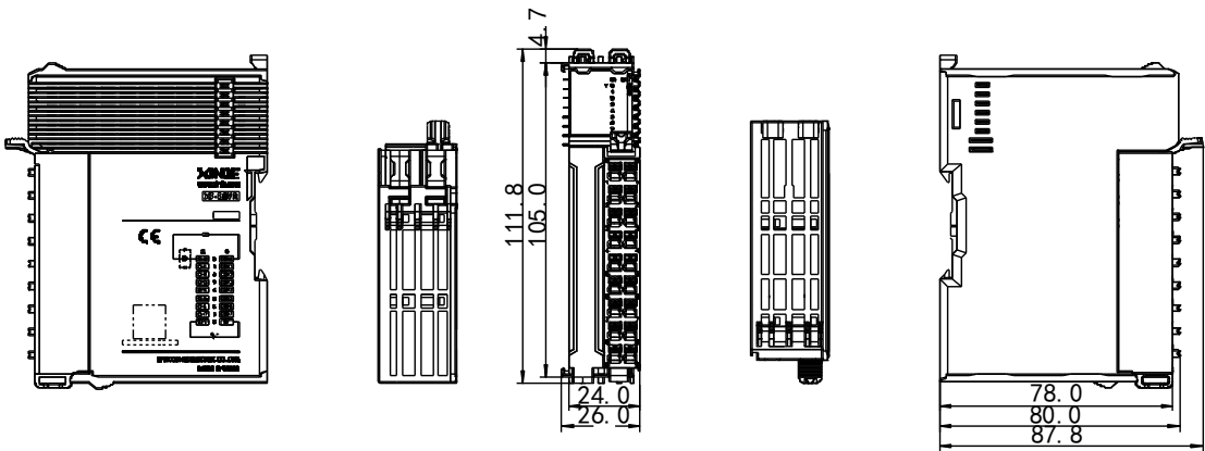
（单位：mm）
