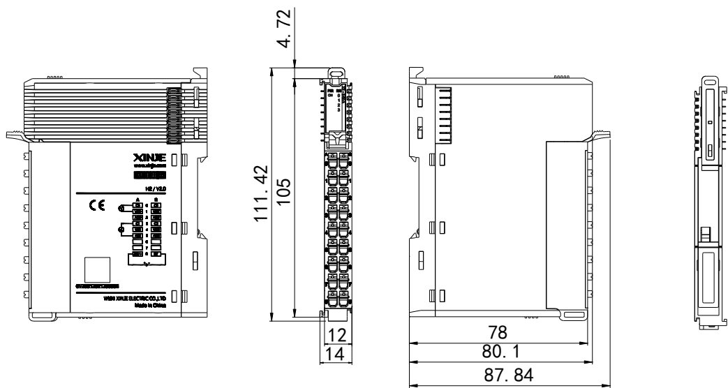
(单位: mm)
