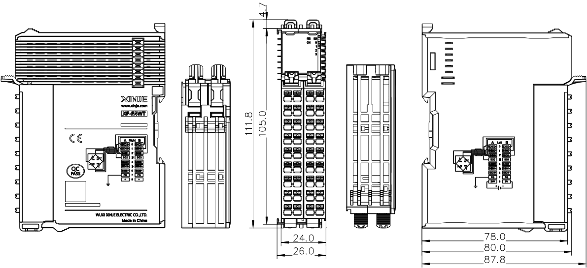
(单位: mm)
