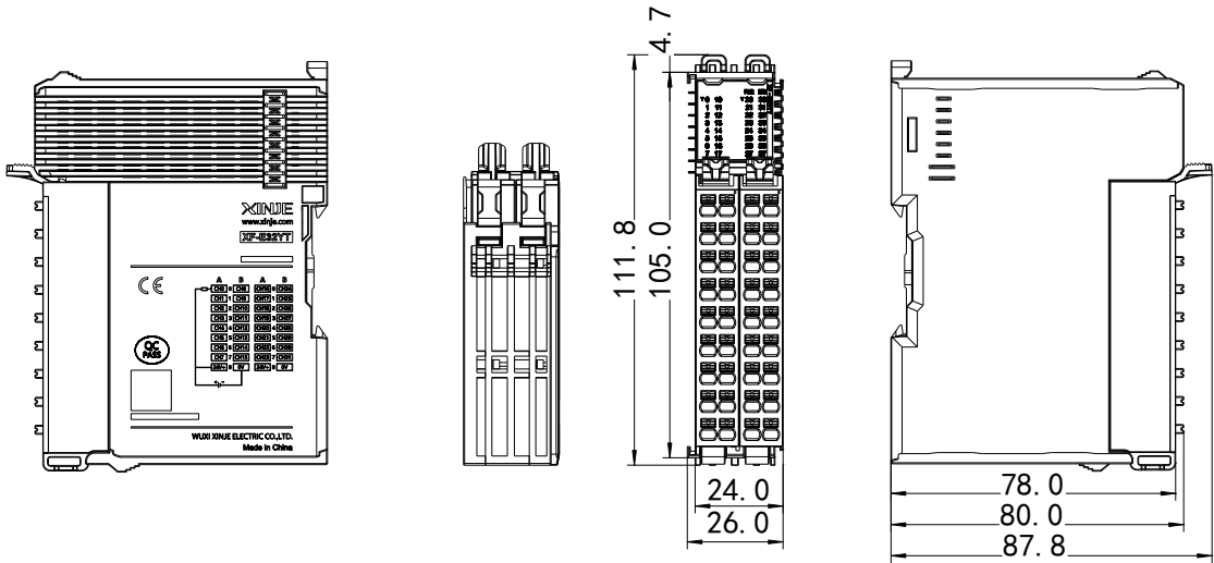
（单位：mm）
