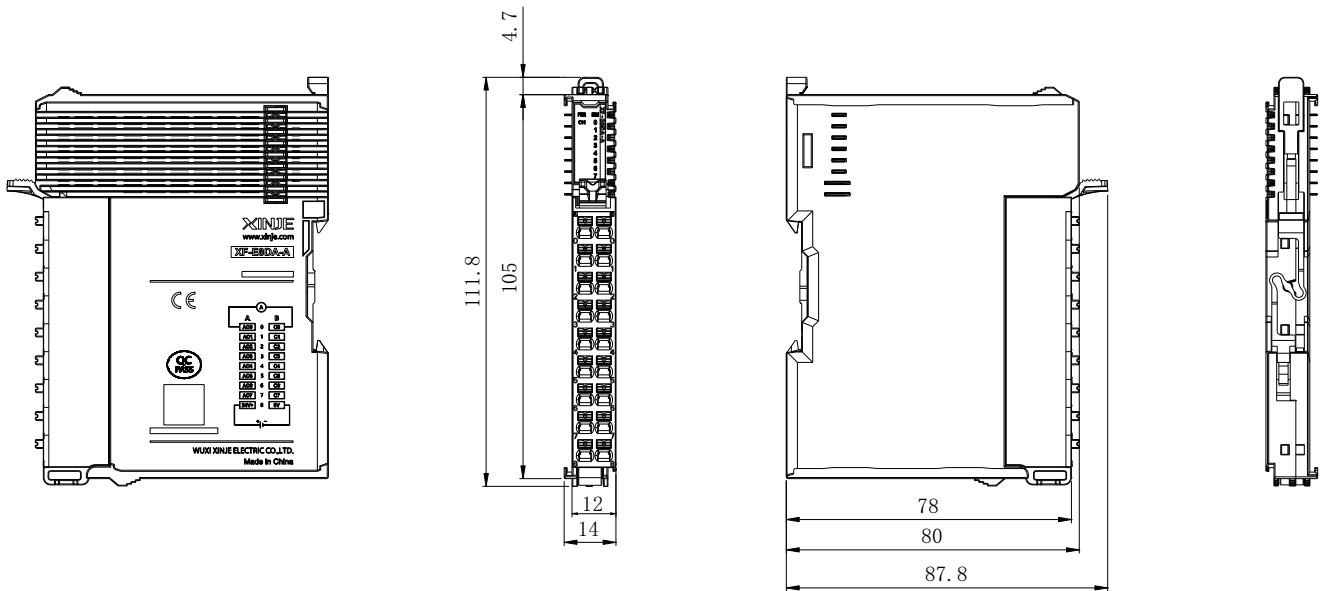
(单位：mm)
