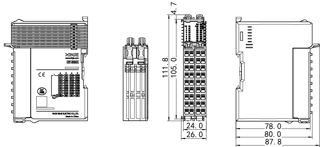
(单位：mm)
