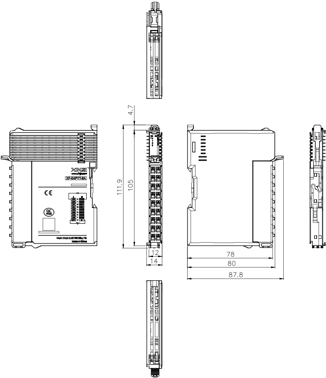
（单位：mm）
