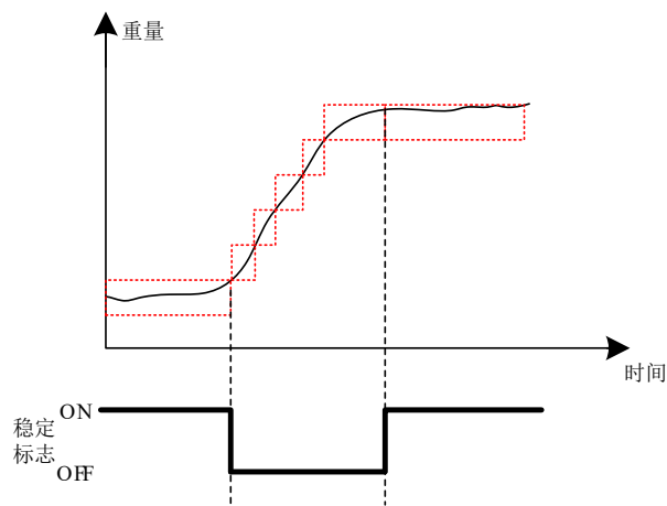
图 3.2 判稳示意图
