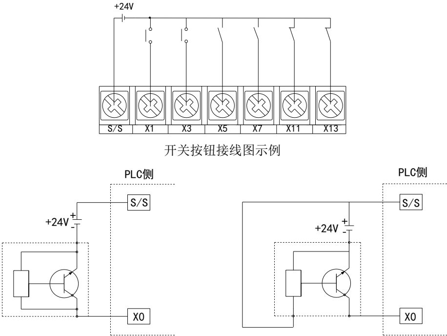
两线制（常开或常闭）接近开关接线图示例 三线制（NPN 型）接近开关接线图示例
