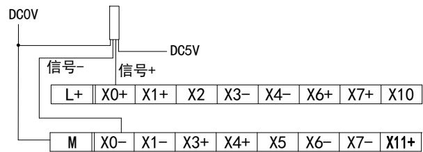
差分接线图示例
