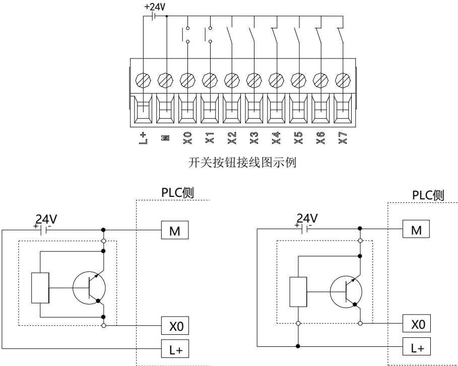
两线制（常开或常闭）接近开关接线图示例 三线制（NPN 型）接近开关接线图示例
