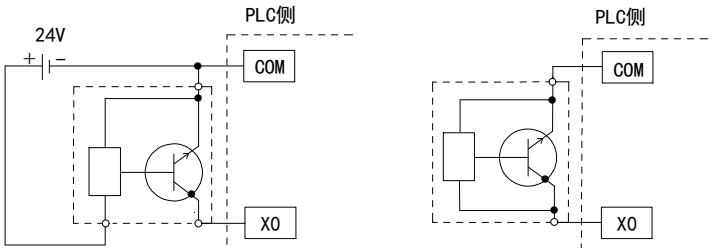
三线制 (NPN 型) 接近开关接线图示例
