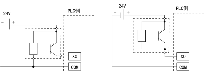
三线制 (PNP 型) 接近开关接线图示例
