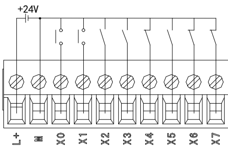
开关按钮接线图示例
