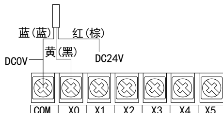
三线制（PNP 型）接近开关接线图示例
